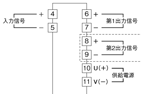
端子接続図
