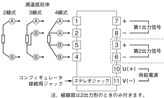
端子接続図
