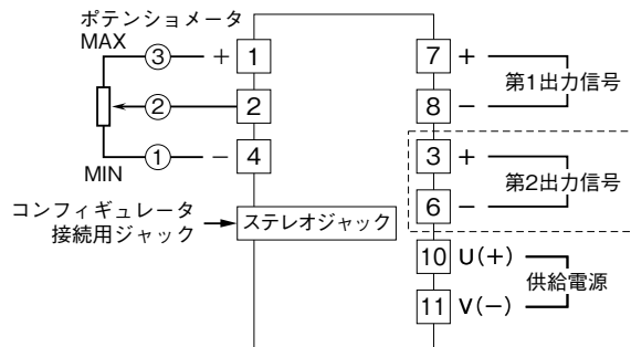
端子接続図
