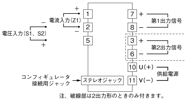
端子接続図
