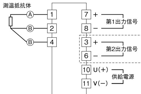
端子接続図
