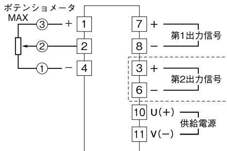
端子接続図
