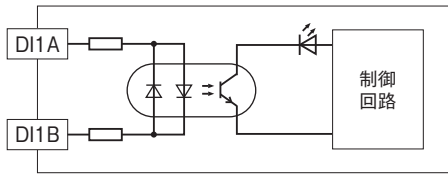
■接点入力回路
