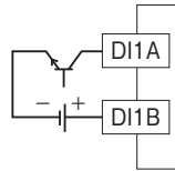
NPN接続
