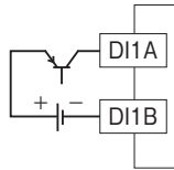
PNP接続
