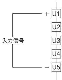
●直流電流 (0~20mA DC)
