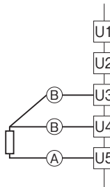
●測温抵抗体および抵抗器 (3線式)
