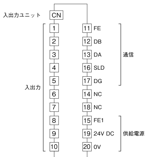
端子接続図
