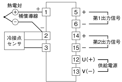
端子番号図
