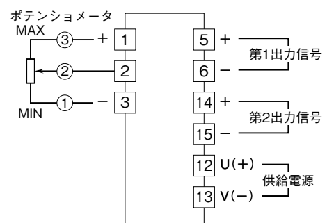
端子接続図
