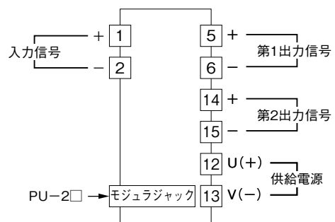
端子接続図
