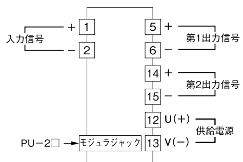
端子接続図
