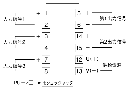
端子接続図
