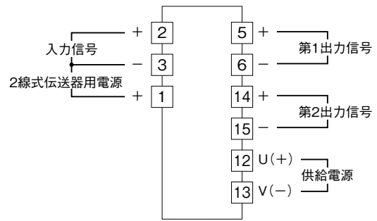
端子接続図
