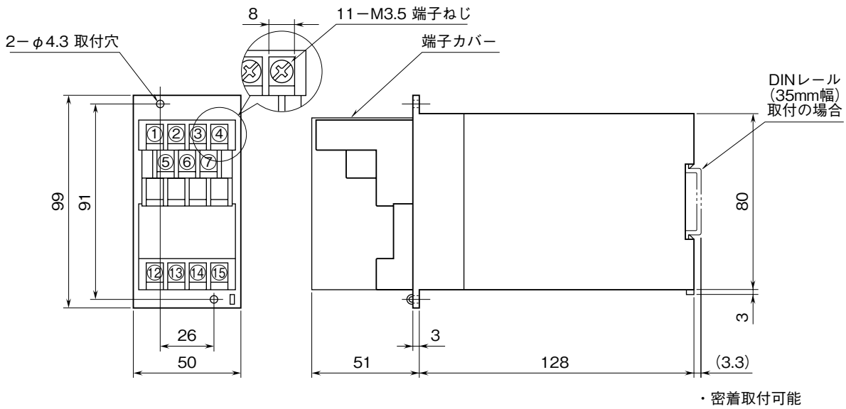
取付寸法図 (単位: mm)
