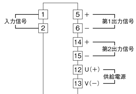
端子接続図
