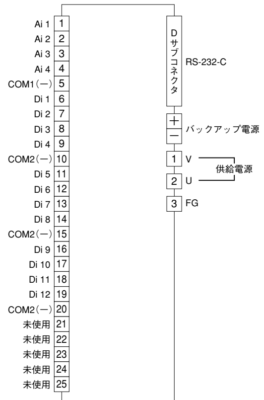
端子接続図
