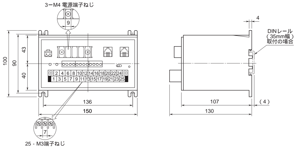
取付寸法図 (単位: mm)
