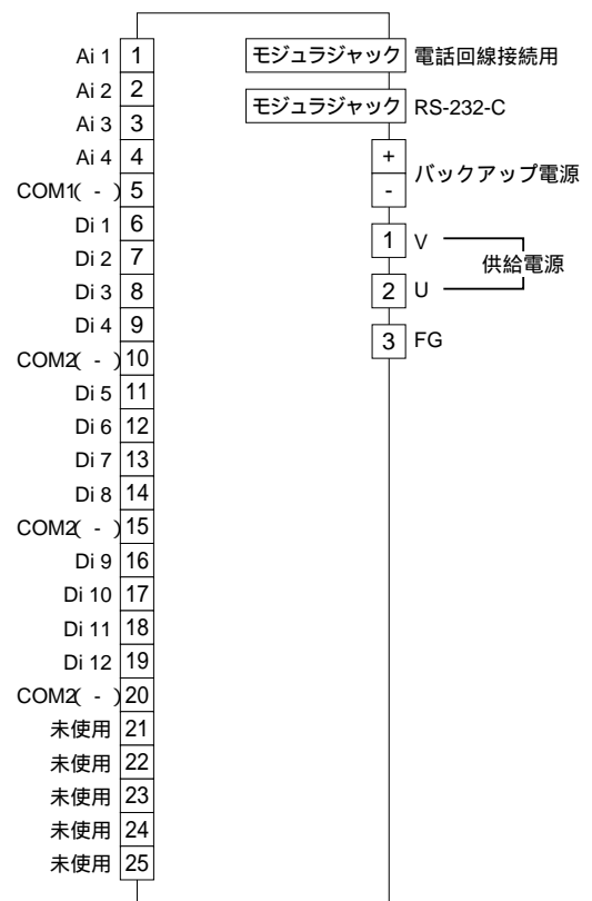
端子接続図
