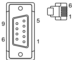
コネクタピン配列
