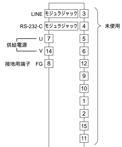
端子接続図
