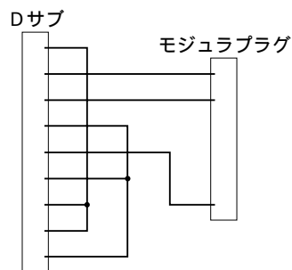
配線図
