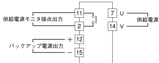
端子接続図
