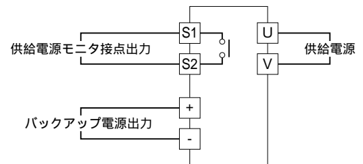
端子接続図
