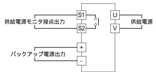
端子接続図
