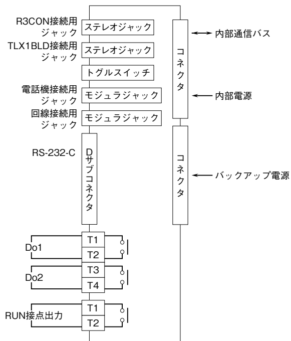
端子接続図
