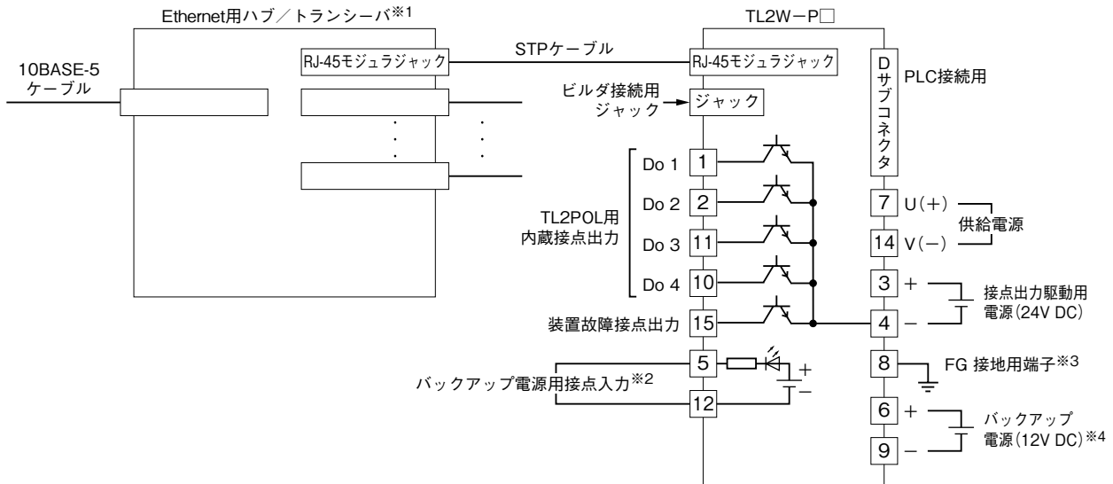
端子接続図
