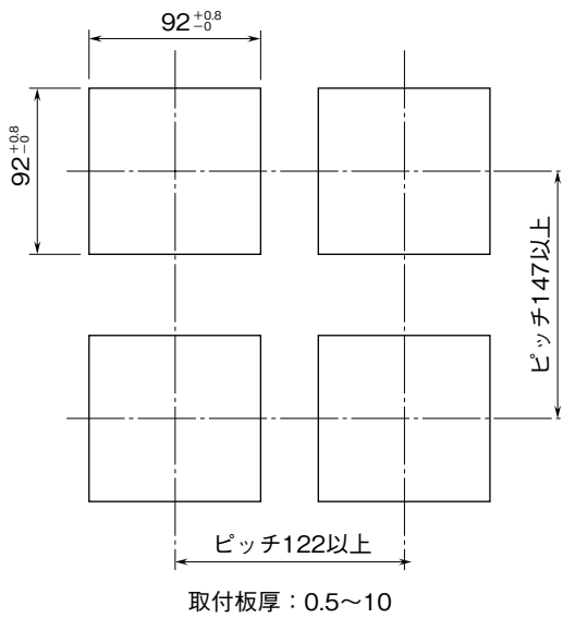
取付寸法図 (単位: mm)
