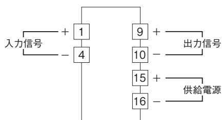
端子接続図
