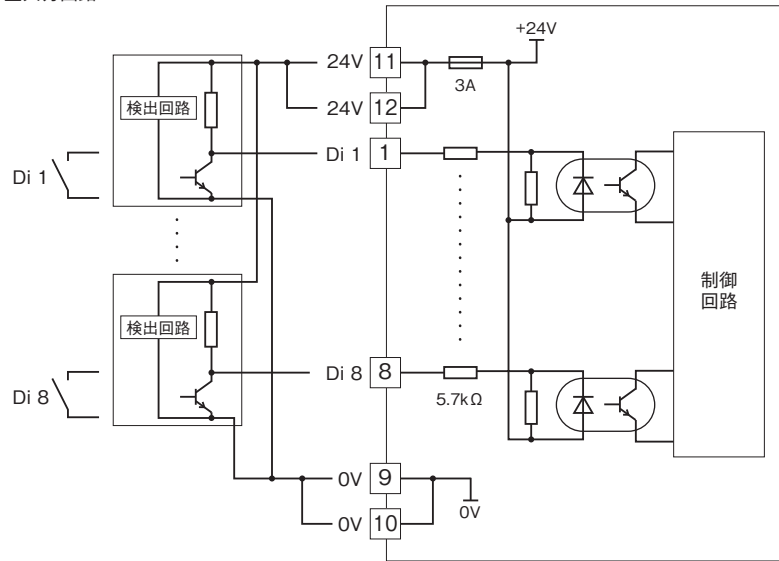
■入力回路
