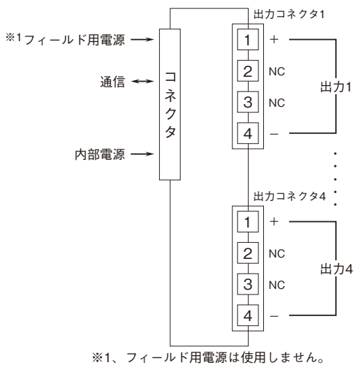
端子接続図
