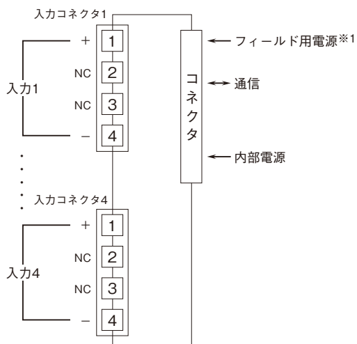
端子接続図
