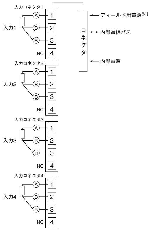
端子接続図
