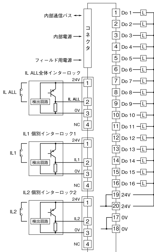
端子接続図
