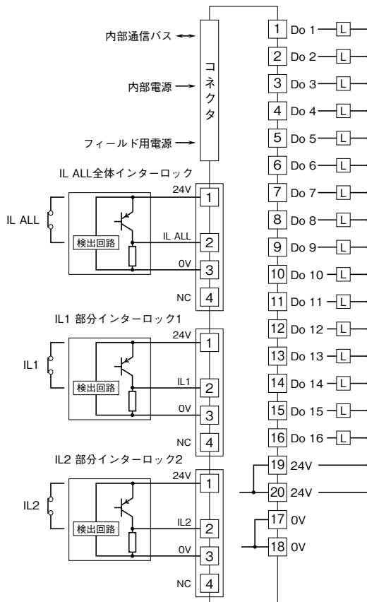
端子接続図
