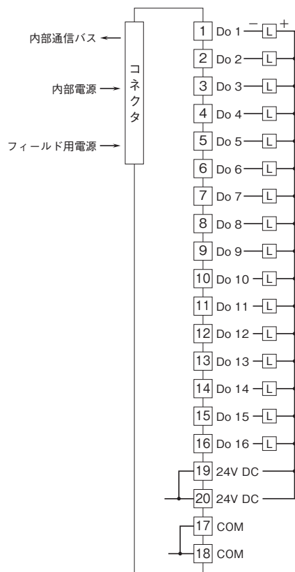
端子接続図
