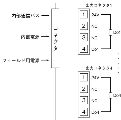
端子接続図
