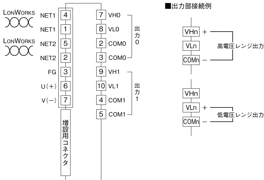
端子接続図
