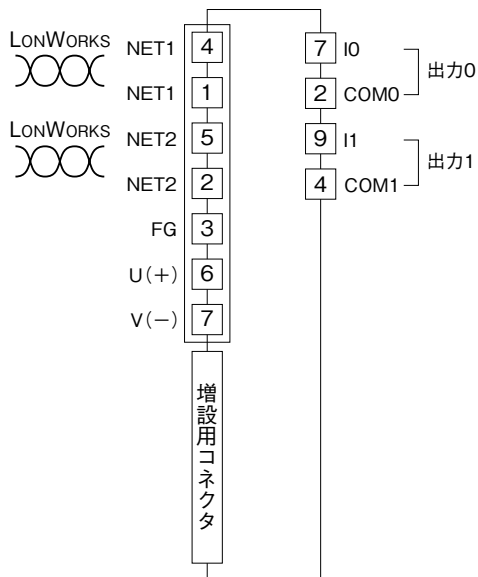
端子接続図
