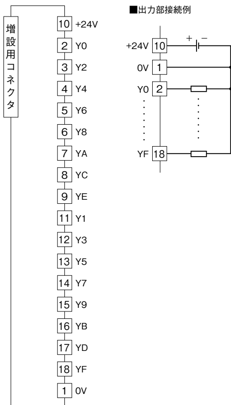
端子接続図
