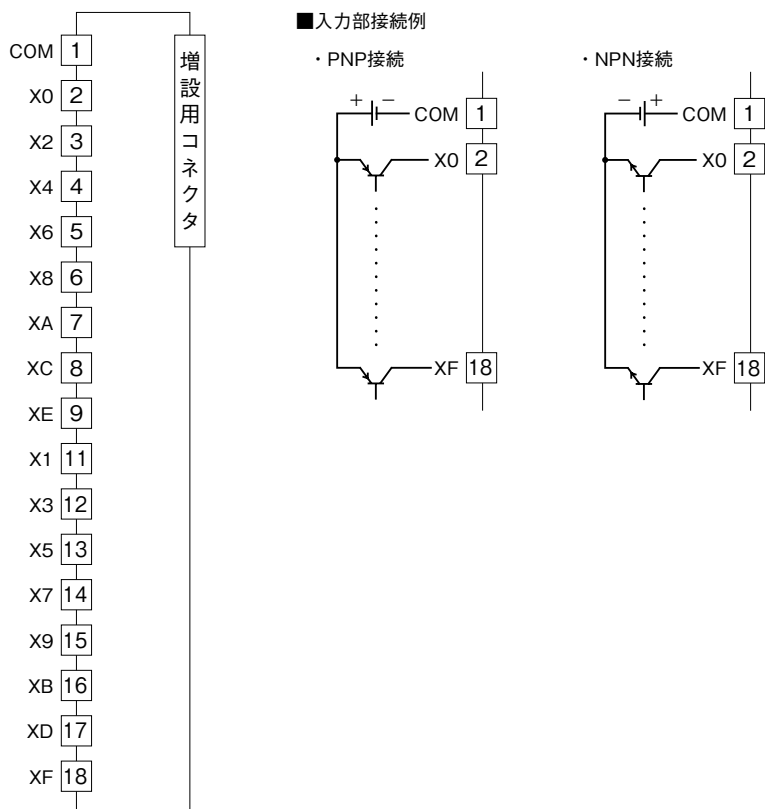
端子接続図
