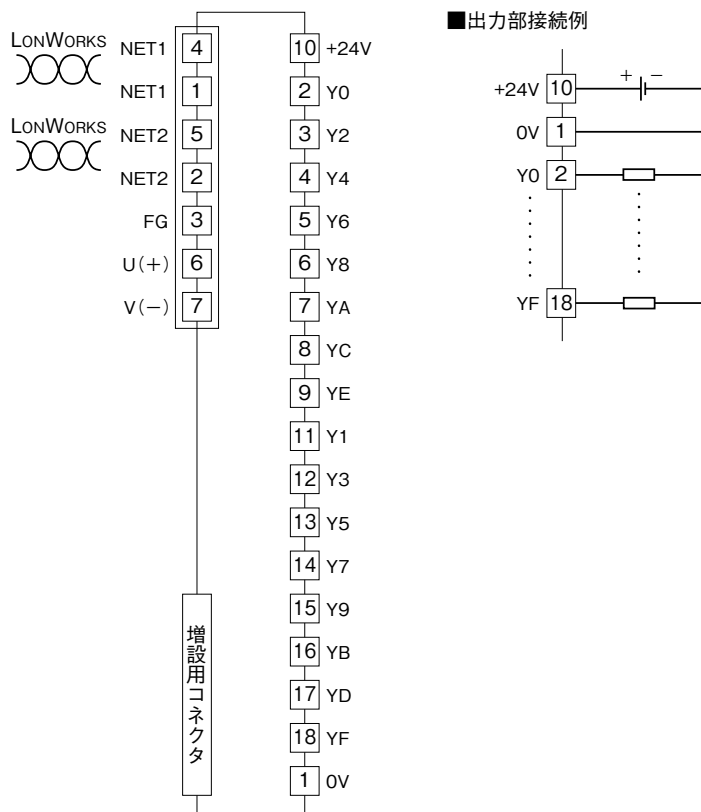
端子接続図
