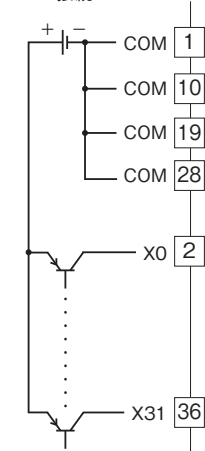
■入力部接続例
