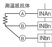
■入力部接続例
