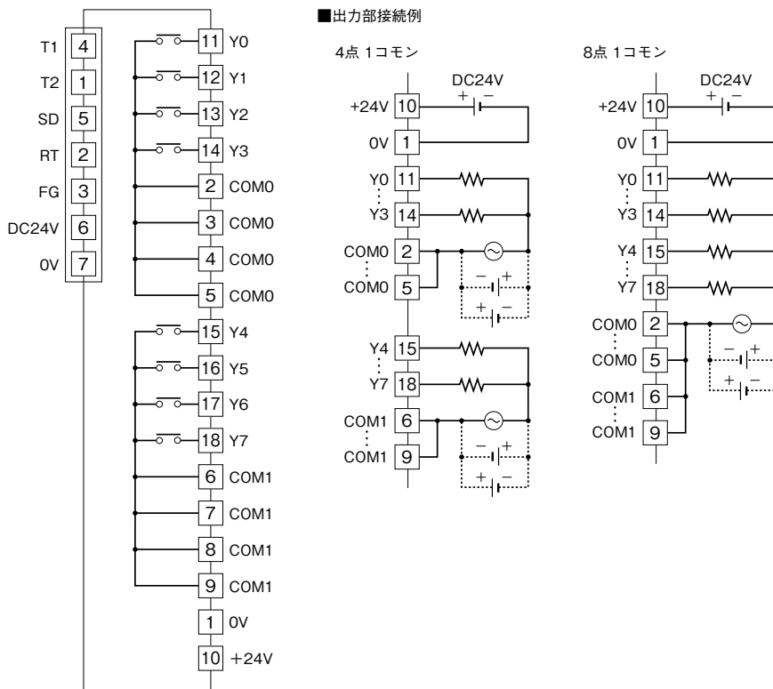
端子接続図
