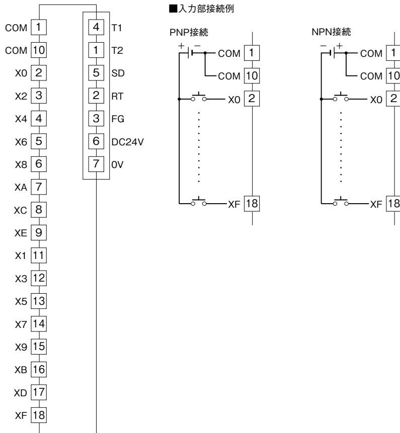
端子接続図
