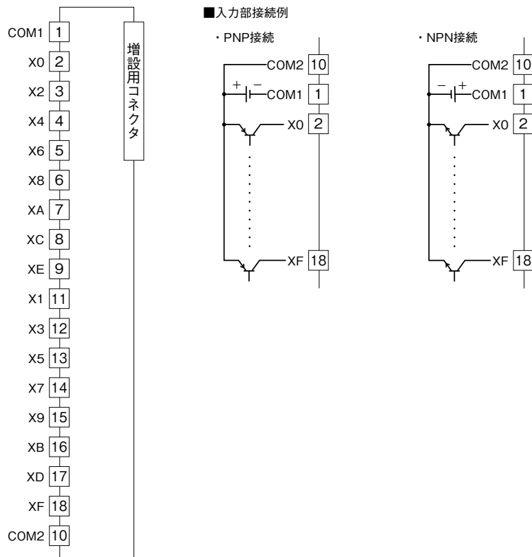
端子接続図
