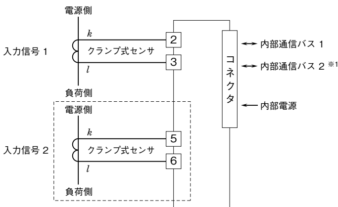
端子接続図
