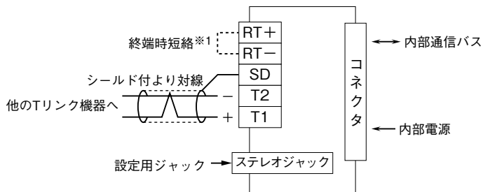
端子接続図
