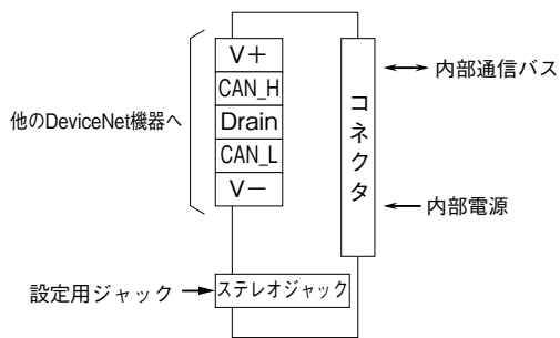
端子接続図
