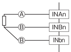
■入力部接続例
