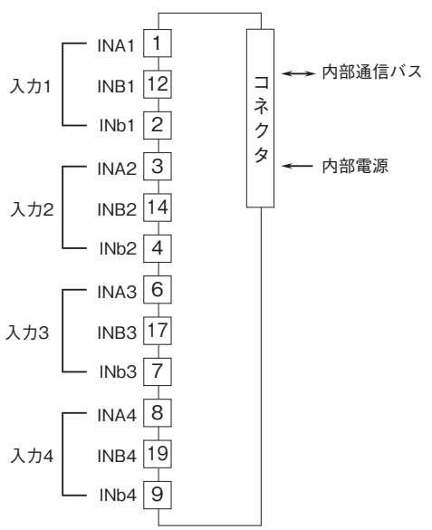
■入力部接続例
