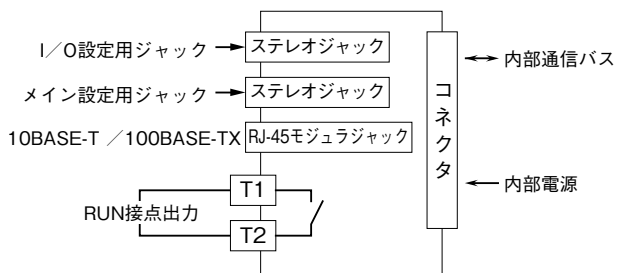
端子接続図
