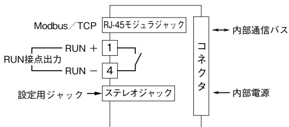
端子接続図
